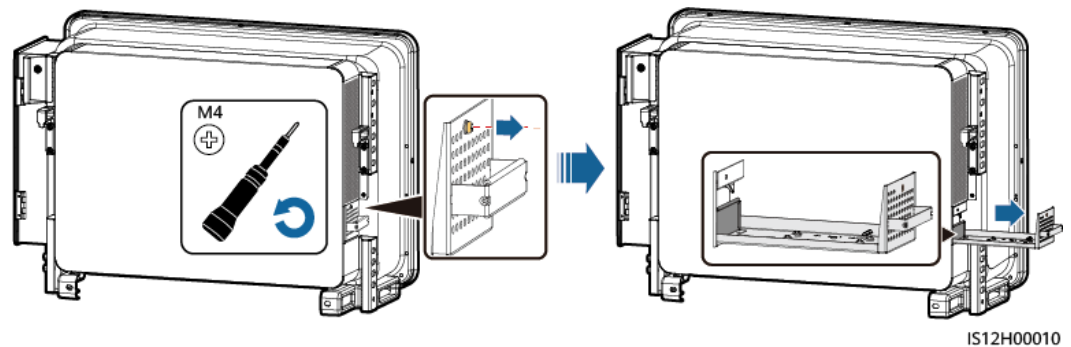
Figura 7-2 Retirando a bandeja do ventilador (1)
