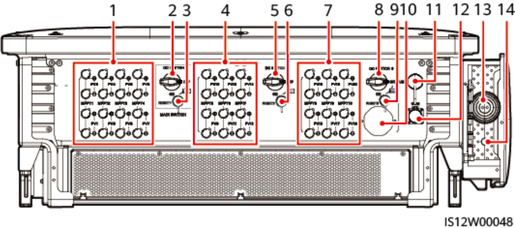
Figura 2-9 Portas
