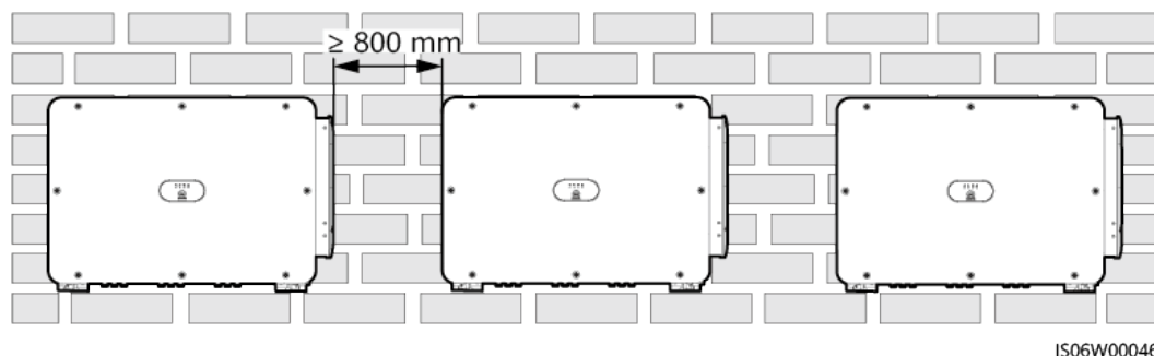
Figura 4-4 Instalação horizontal (recomendada)
