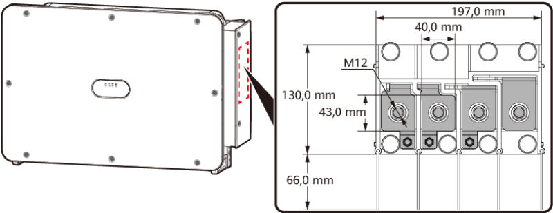
Figura 5-10 Portas de fiação
