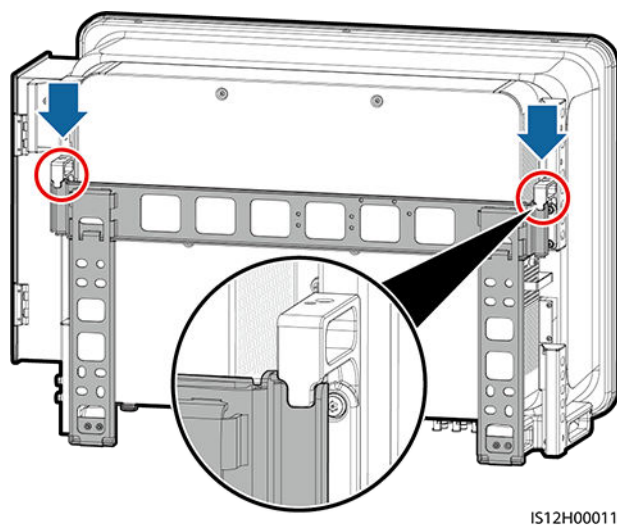
Figura 4-16 Montagem do inversor
