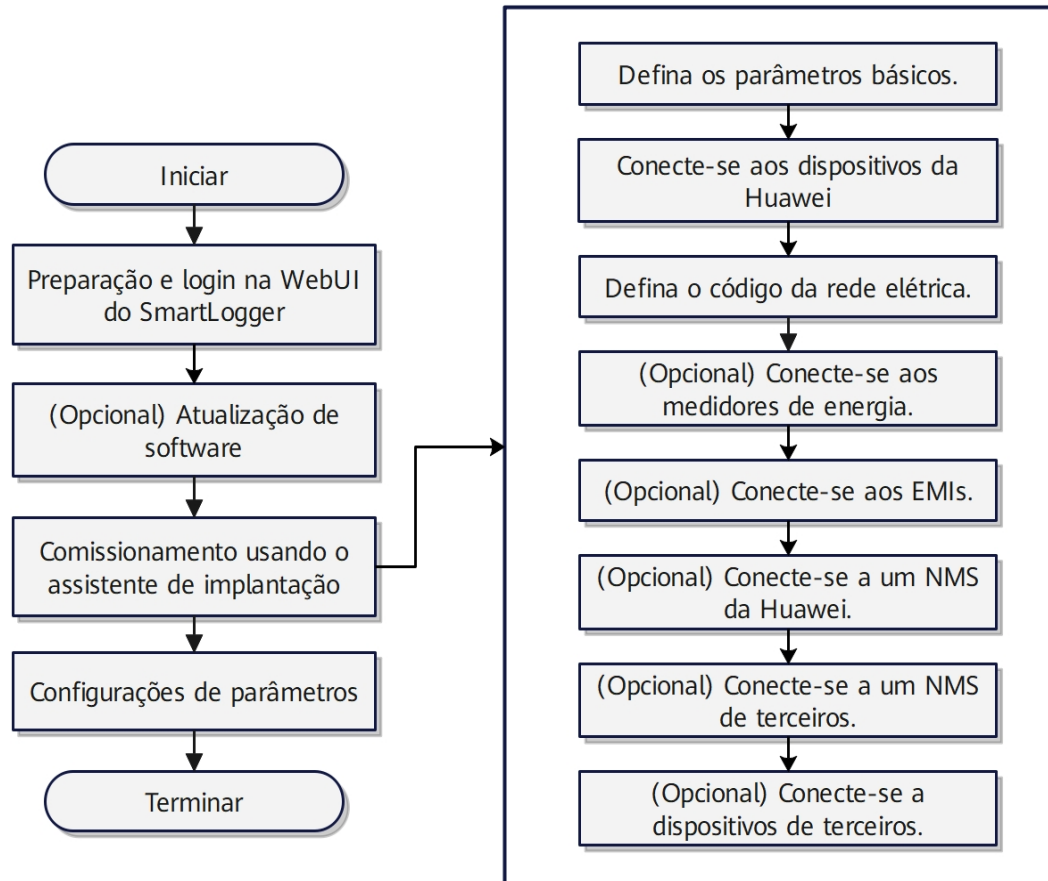
Figura 6-1 Processo de comissionamento na UI da Web do SmartLogger
