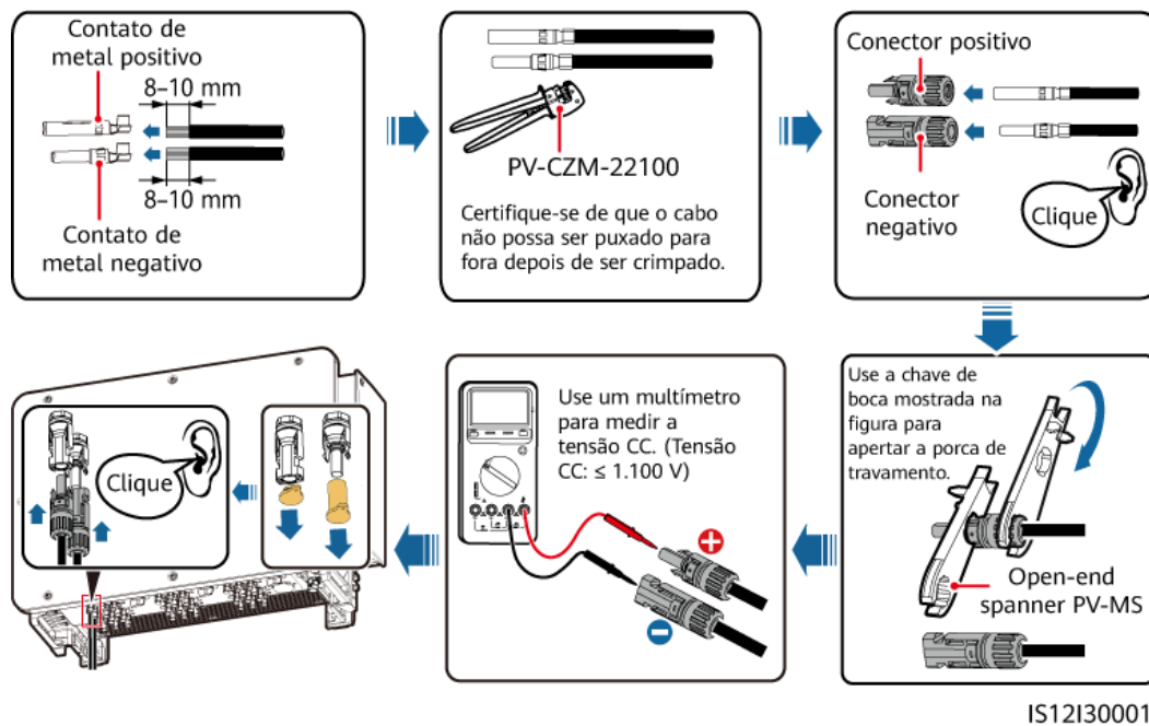
Figura 5-25 Conexão dos cabos de alimentação de entrada CC
