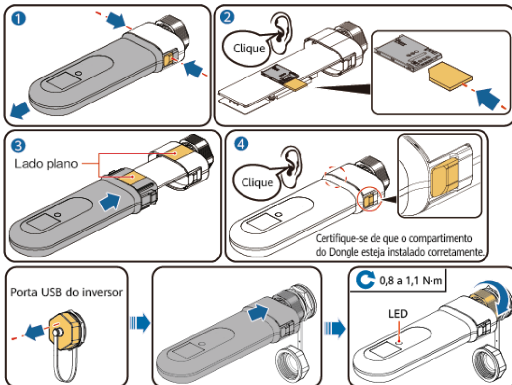
Figura 5-32 Instalação do Smart Dongle 4G (SDongleB-06)
