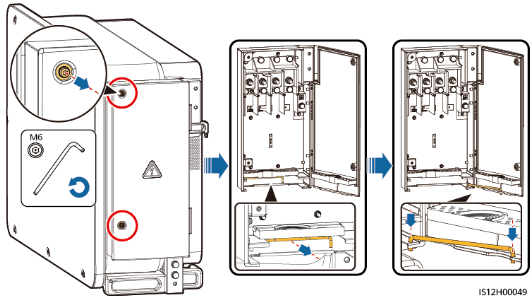
Figura 5-3 Abertura da porta do compartimento de manutenção
