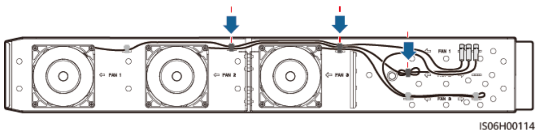
Figura 7-11 Ligando os cabos do FAN 2
