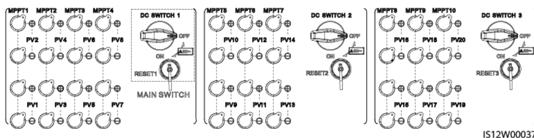
Figura 5-16 Terminais CC
