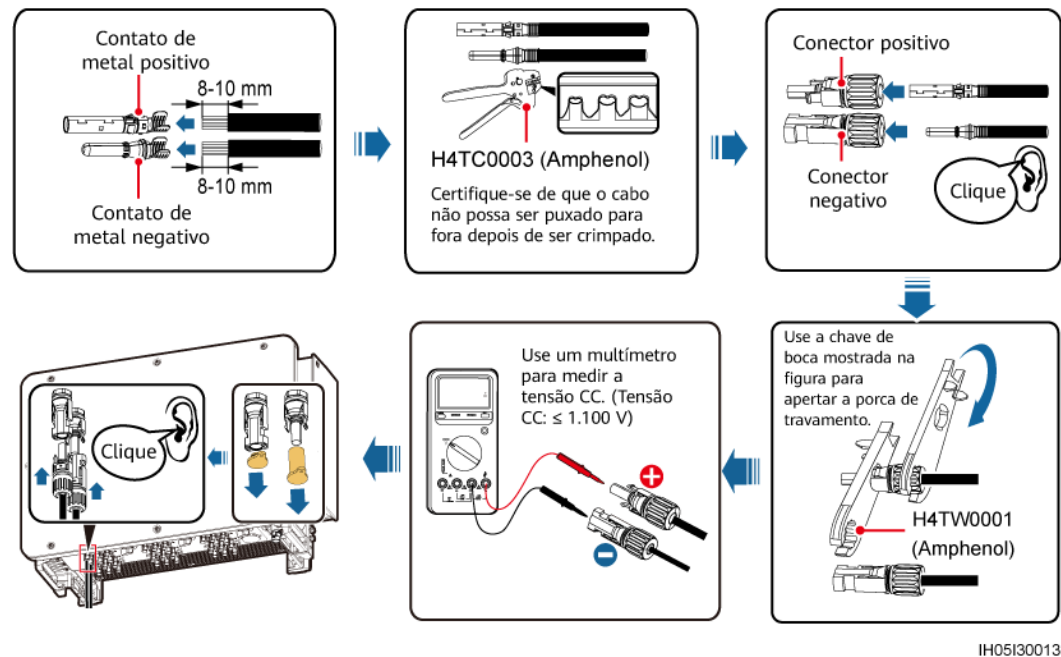
Figura 5-21 Conexão dos cabos de alimentação de entrada CC
