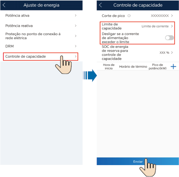
Figura 6-11 Feed-in em corrente limitada
