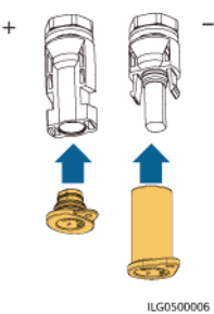
Figura 5-28 Plugues de vedação
