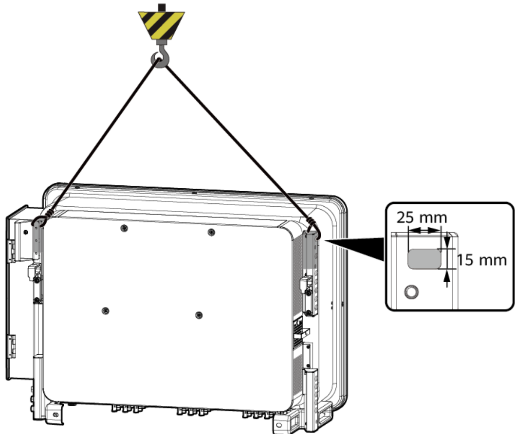
Figura 4-15 Içamento do inversor
