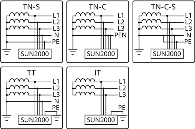
Figura 2-7 Sistemas de aterramento
