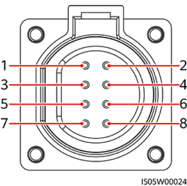
Figura 5-29 Porta de comunicação
