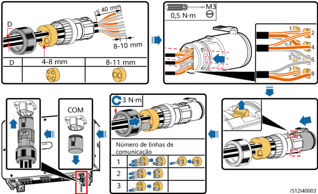
Figura 5-30 Conexão de cabos de comunicação RS485 (anel de borracha de quatro furos de 4–8 mm)
