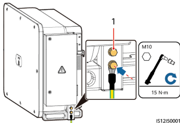
Figura 5-2 Conexão de cabo de PE ao ponto de PE (no invólucro)
