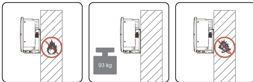
Figura 4-1 Estrutura de montagem
