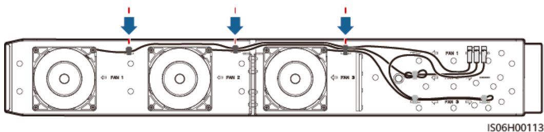
Figura 7-10 Ligando os cabos do FAN 1
