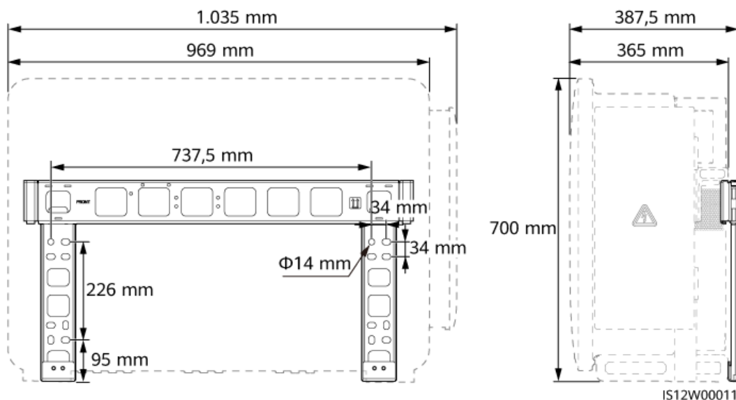
Figura 2-10 Dimensões
