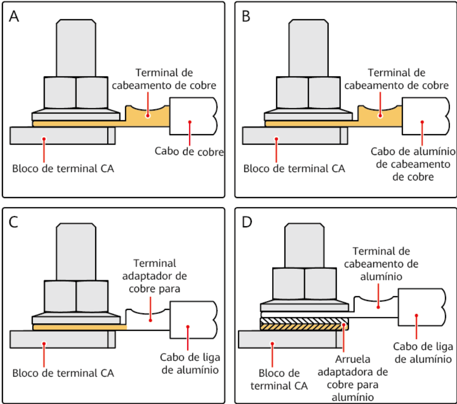
Figura 5-9 Requisitos para o terminal OT/DT
