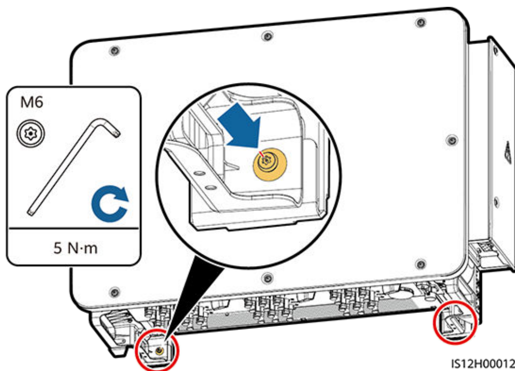
Figura 4-17 Aperto dos parafusos de segurança Torx
