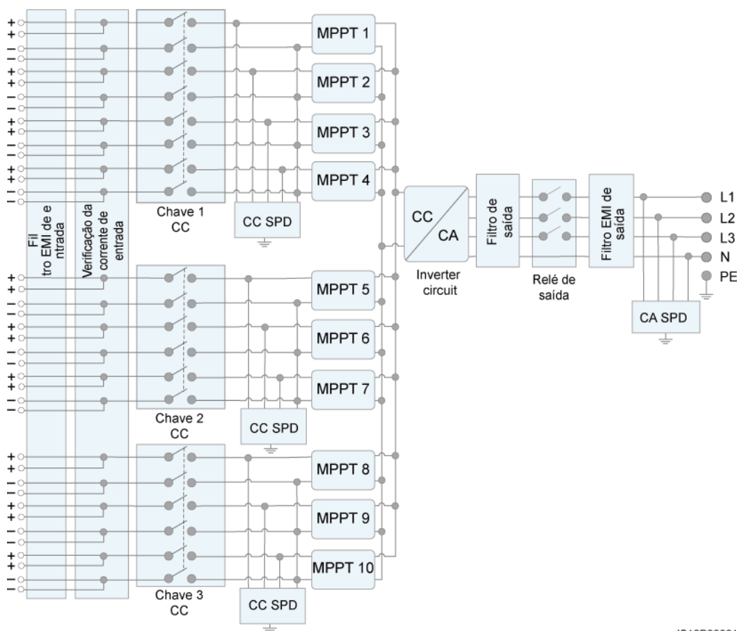
Figura 2-13 Diagrama esquemático
