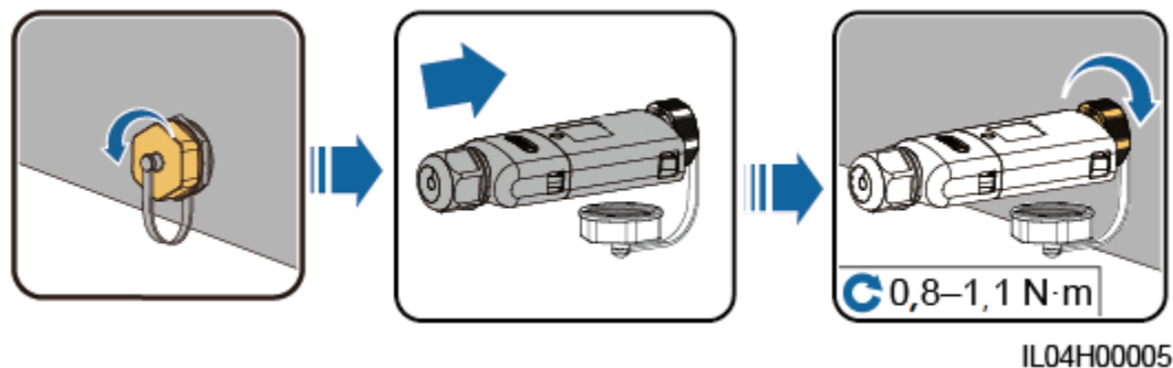
Figura 5-33 Instalação do Smart Dongle WLAN-FE (SDongleA-05 para o cenário de comunicação por WLAN)
