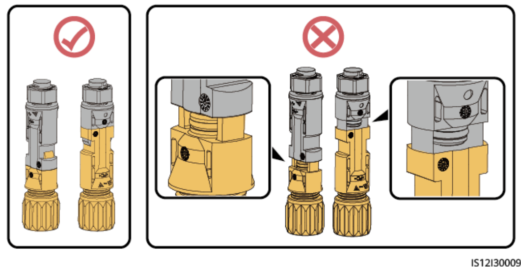
Figura 5-22 Conexão do conector
