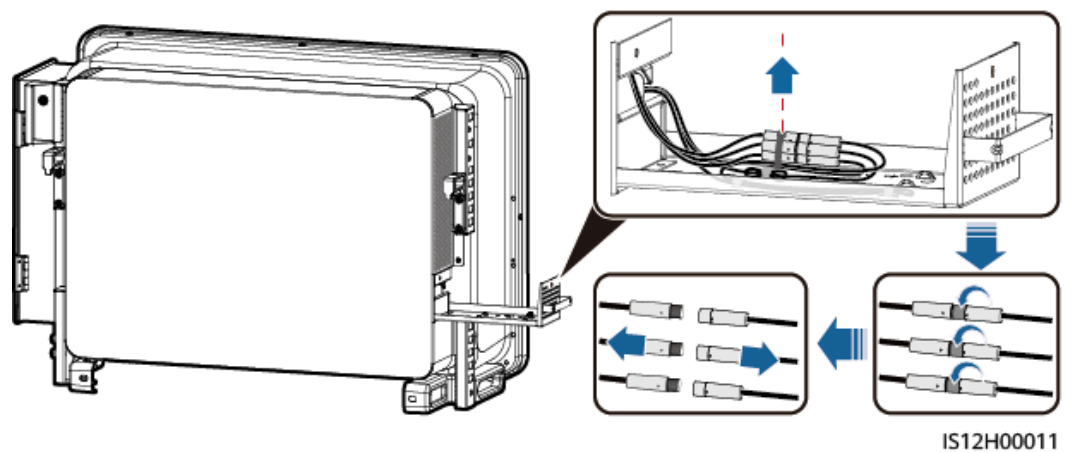
Figura 7-3 Desconectando os cabos
