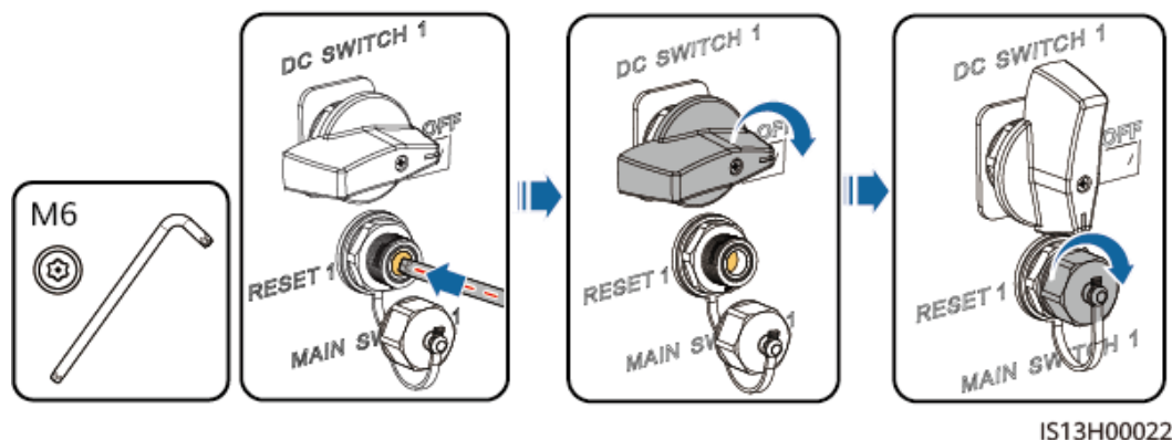
Figura 7-16 Redefinição e inicialização do interruptor CC (o DC SWITCH 1 é usado como exemplo)
