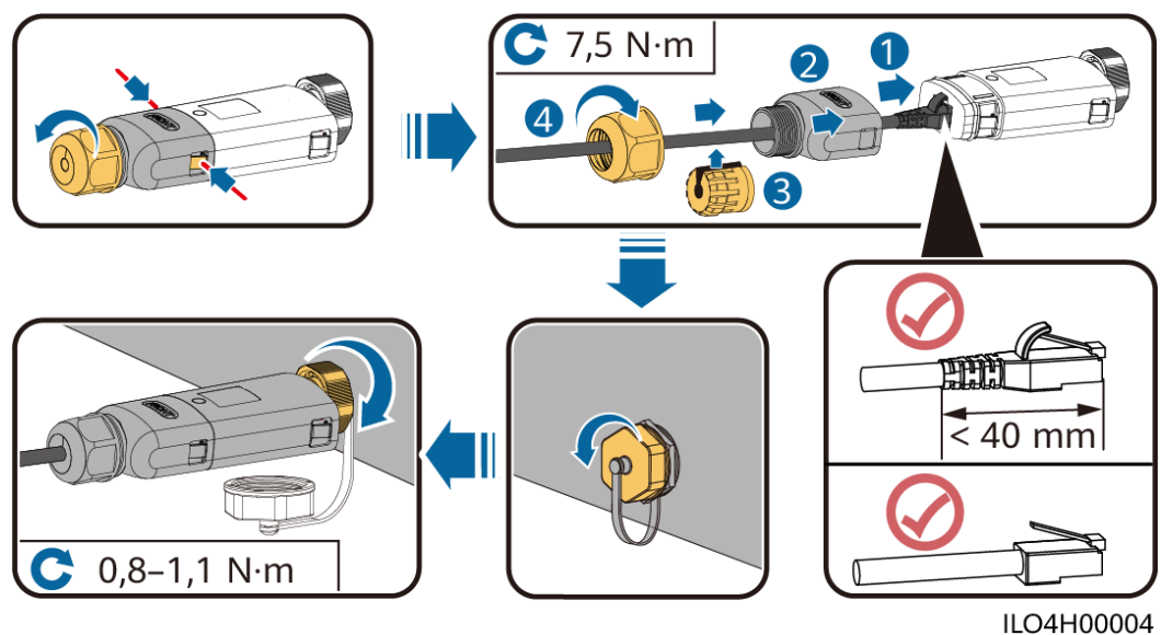
Figura 5-34 Instalação do Smart Dongle WLAN-FE (SDongleA-05 para o cenário de comunicação por FE)
