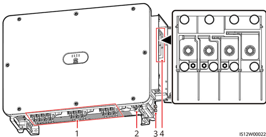
Figura 2-11 Portas de fiação
