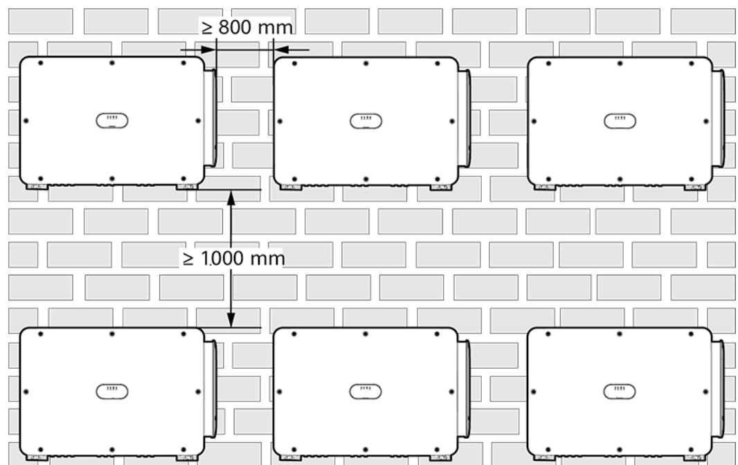
Figura 4-6 Instalação empilhada (não recomendada)
