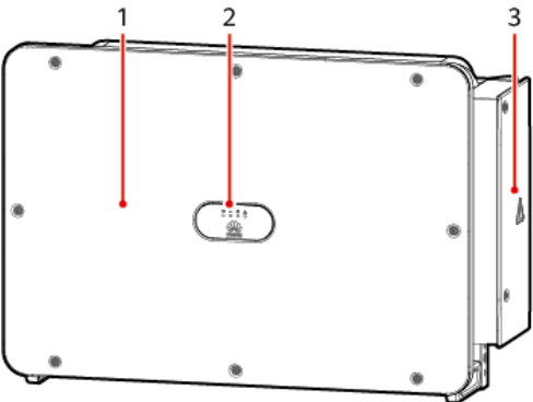
Figura 2-8 Vista frontal
