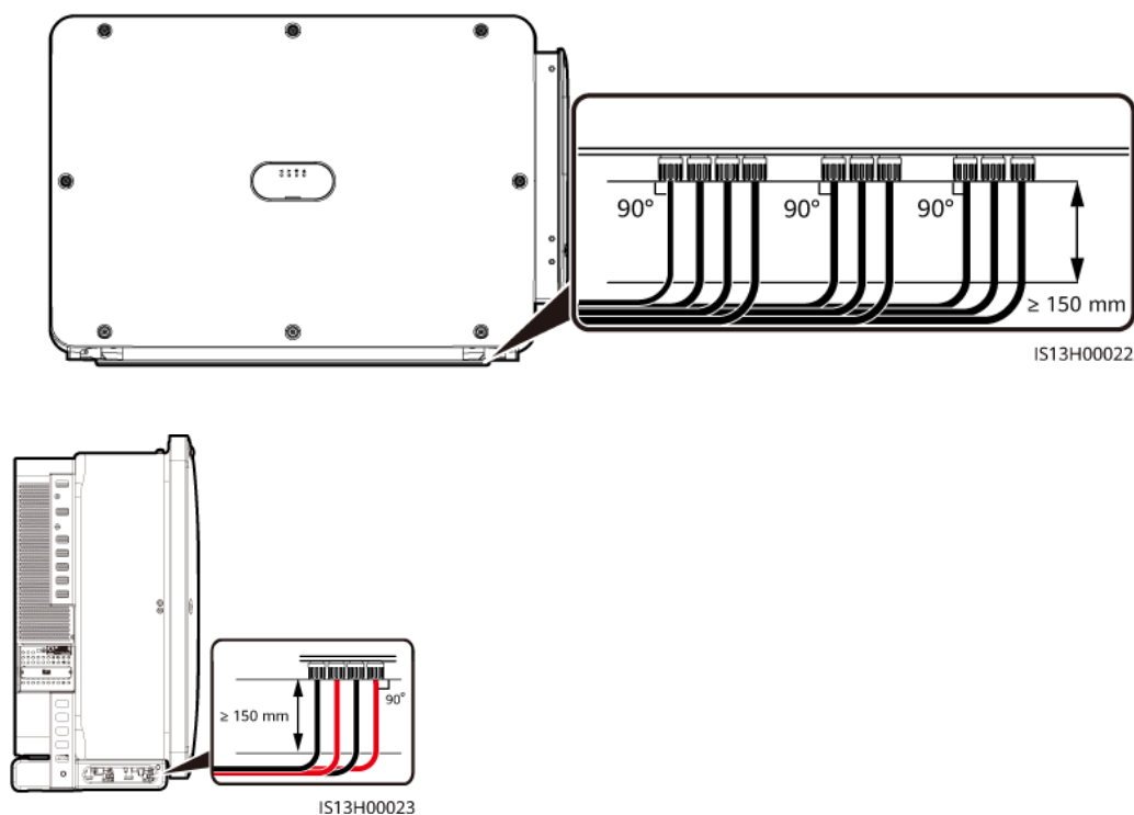
Figura 5-23 Requisitos de cabeamento de alimentação de entrada CC
