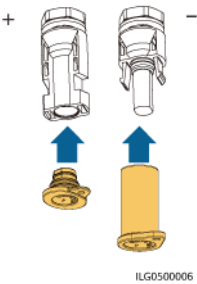
Figura 5-24 Plugues de vedação
