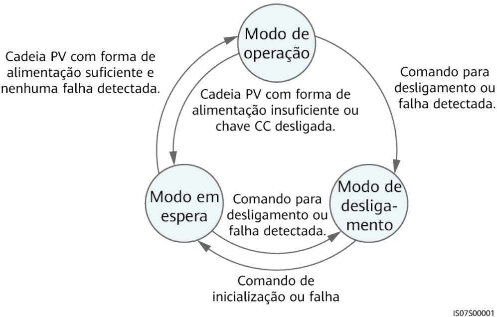
Figura 2-14 Modos de funcionamento
