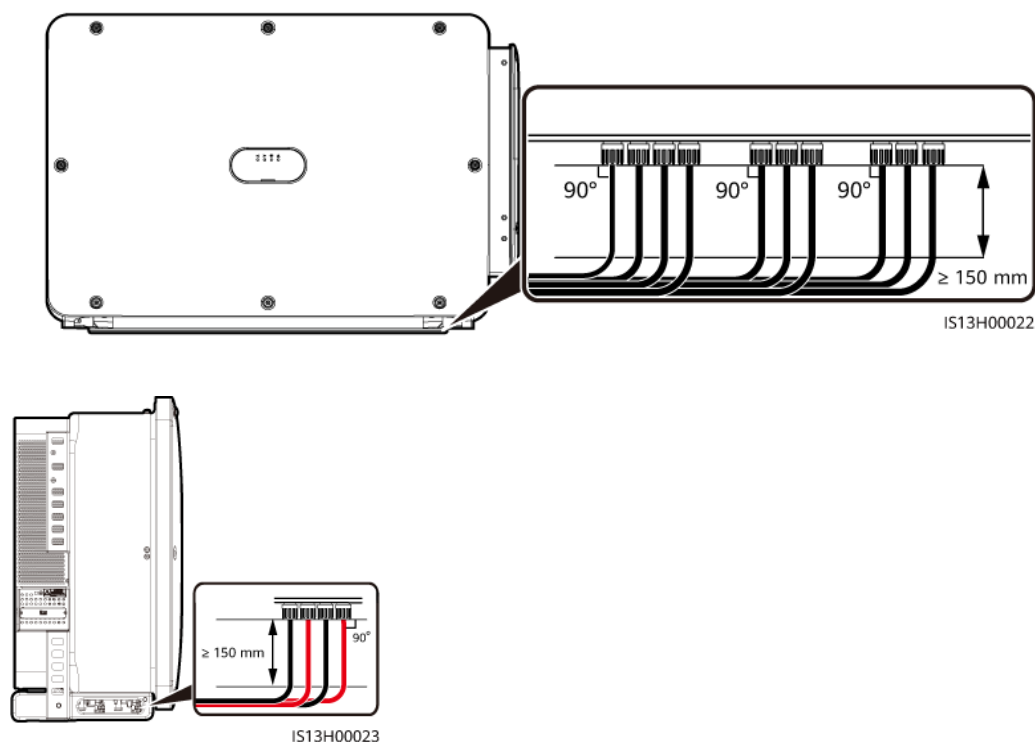
Figura 5-27 Requisitos de cabeamento de alimentação de entrada CC
