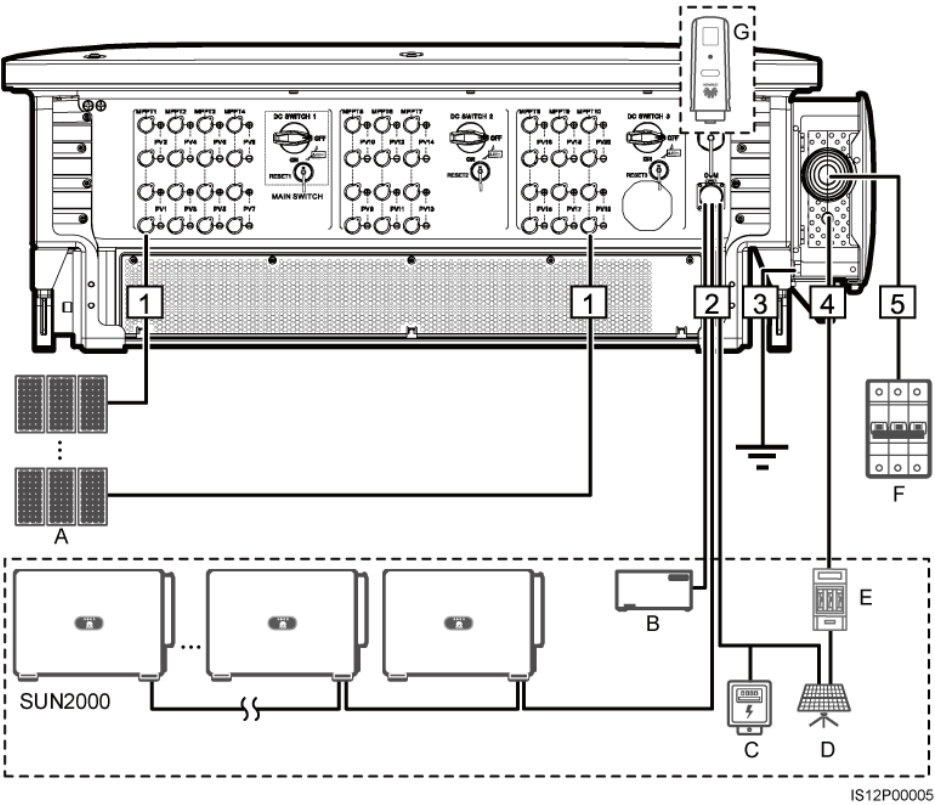
Figura 5-1 Conexões de cabos do inversor (configure os componentes na caixa pontilhada conforme necessário)
