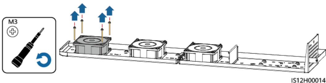
Figura 7-8 Removendo um ventilador
