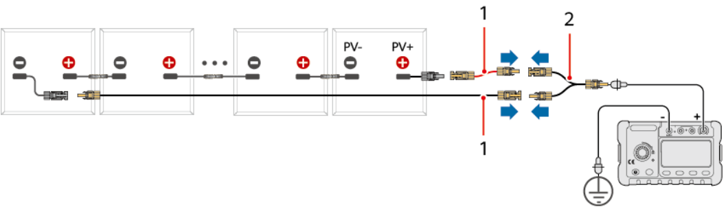
Figura 5-20 Medição da resistência de isolamento do cabo de extensão
