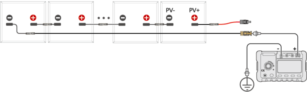
Figura 5-18 Medição da resistência de isolamento do FV– para cada cadeia FV
