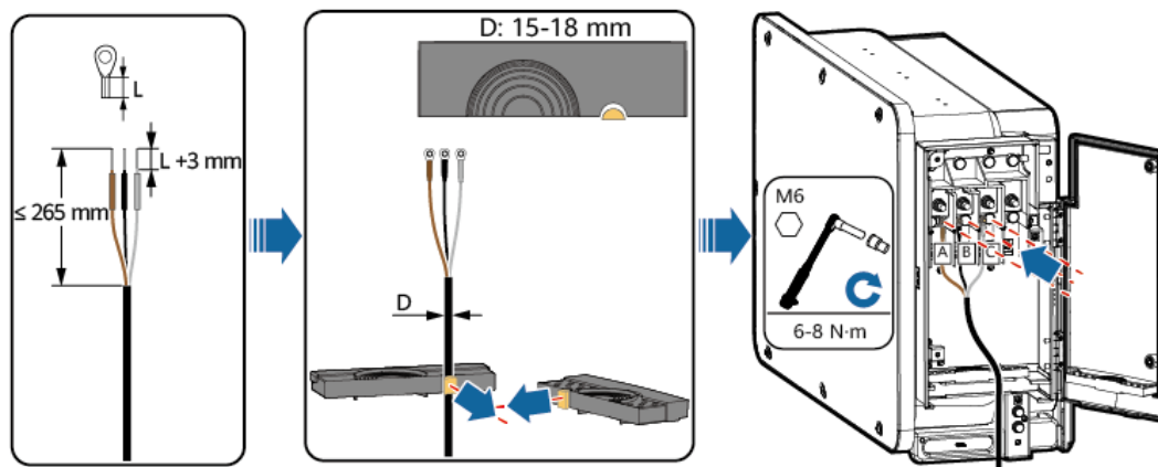
Figura 5-7 Conexão do cabo de alimentação do sistema de rastreamento
