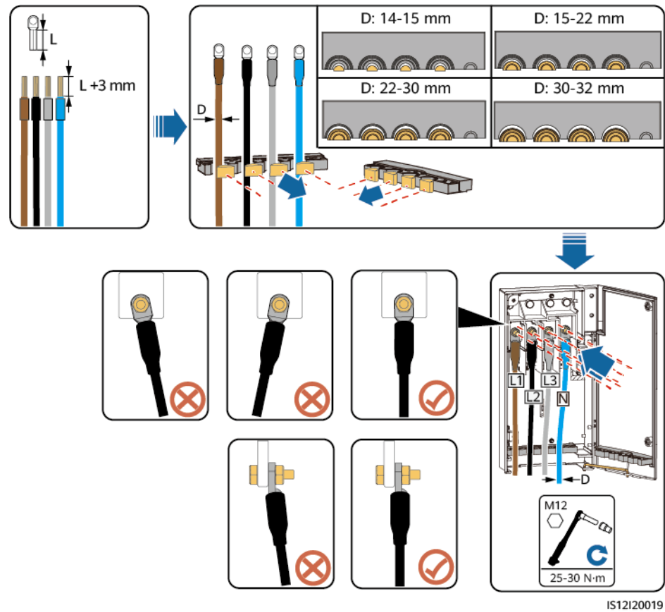
Figura 5-13 Conexão de cabo de núcleo único
