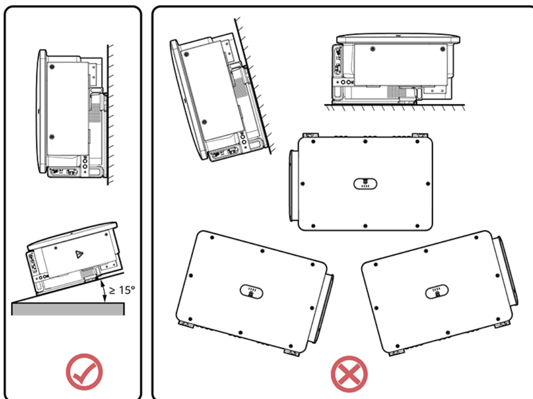
Figura 4-2 Ângulo de instalação
