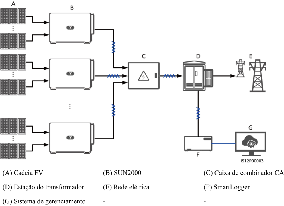
Figura 2-5 Rede do MBUS (SmartLogger)
