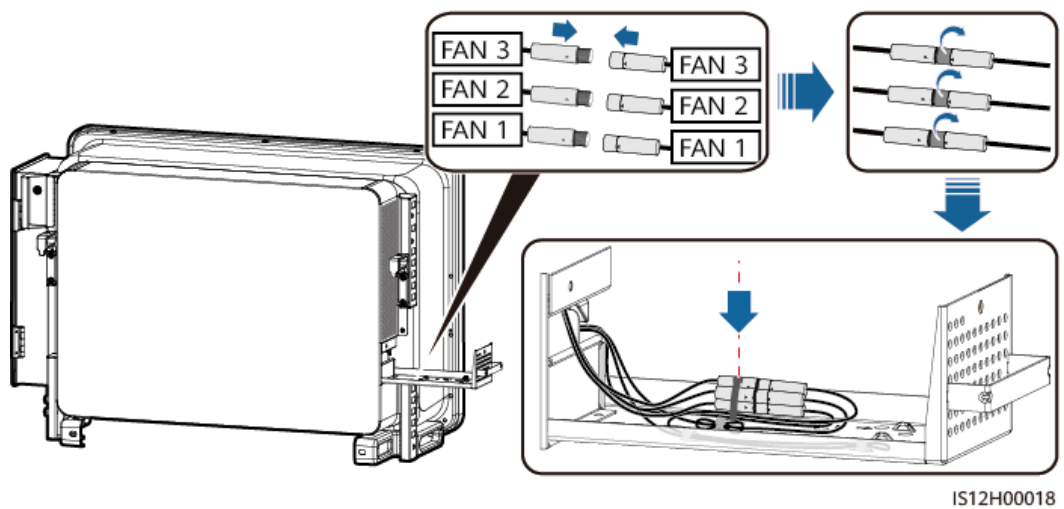
Figura 7-14 Prendendo os cabos
