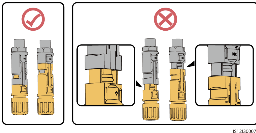
Figura 5-26 Conexão do conector
