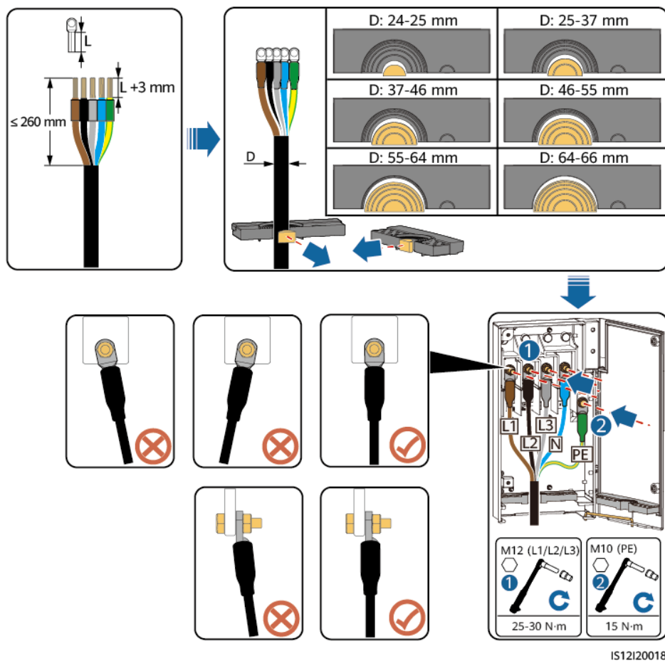
Figura 5-12 Conexão de cabo de vários núcleos
