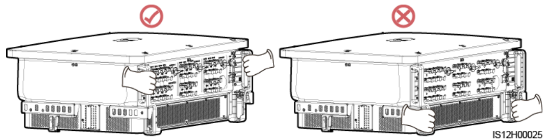
Figura 4-12 Posições de elevação
