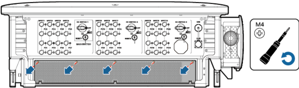
Figura 7-1 Removendo a placa defletora do orifício de entrada de ar
