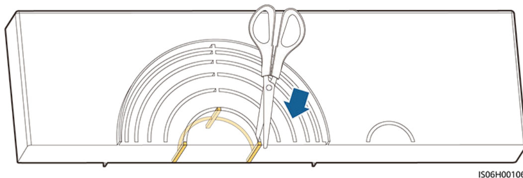
Figura 5-6 Remoção de um anel de borracha
