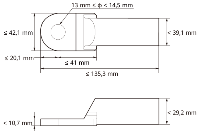
Figura 5-11 Especificações do terminal OT/DT crimpado
