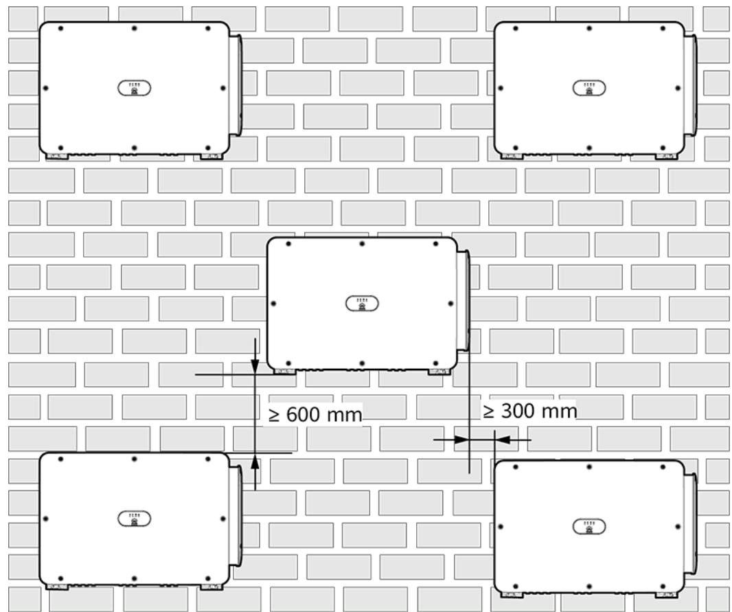
Figura 4-5 Instalação triangular (recomendada)
