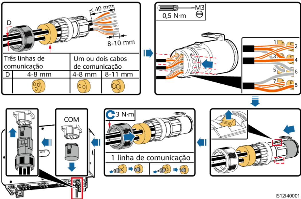
Figura 5-31 Conexão de cabos de comunicação RS485 (anel de borracha de dois ou três furos de 4–8 mm)
