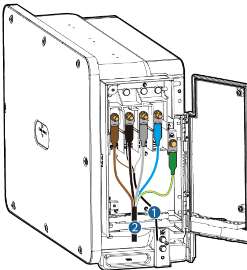
Figura 5-8 Sequência de conexão do cabo
