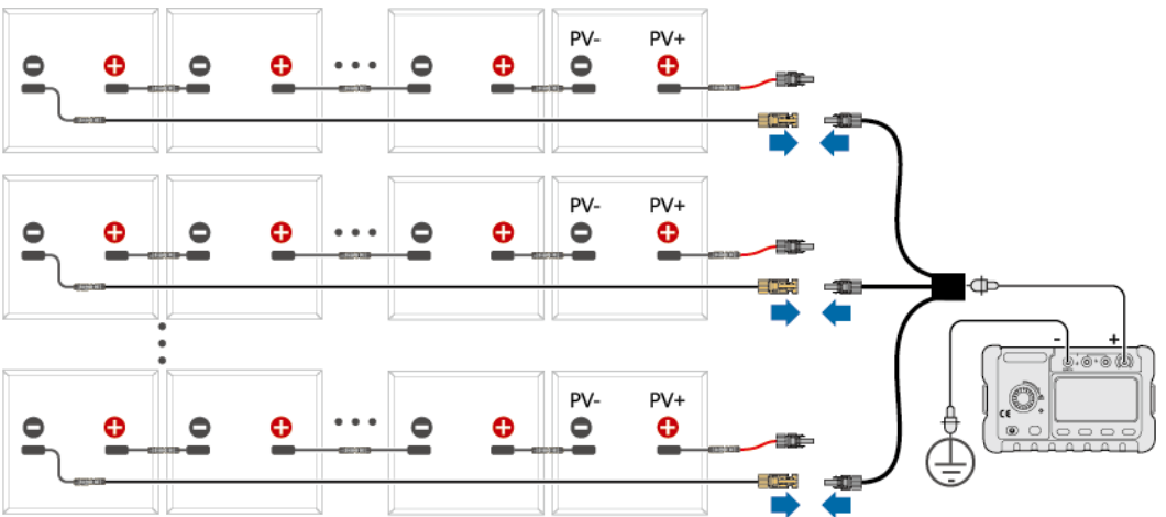
Figura 5-19 Medição da resistência de isolamento de FV– para todas as cadeias FV
