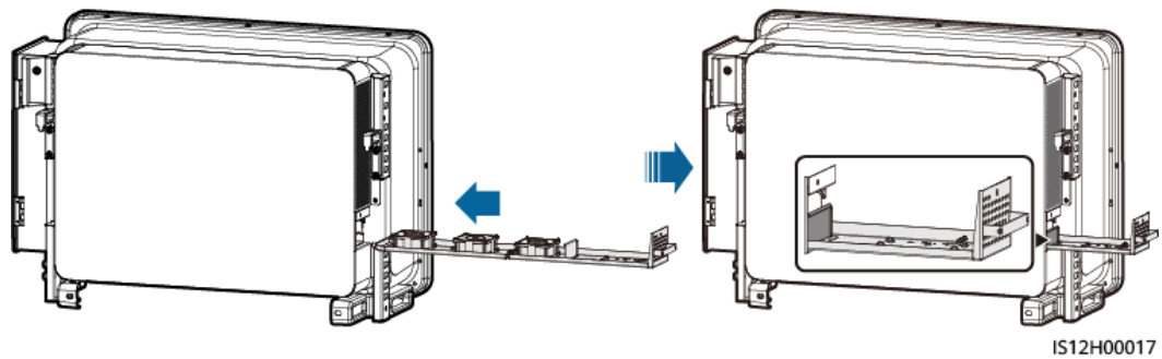
Figura 7-13 Empurrando a bandeja do ventilador
