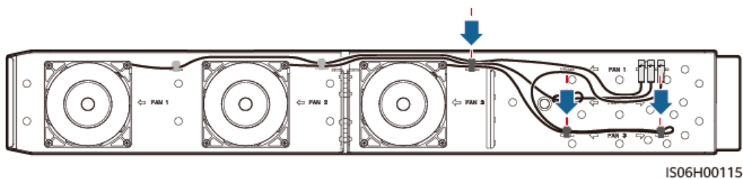
Figura 7-12 Ligando os cabos do FAN 3
