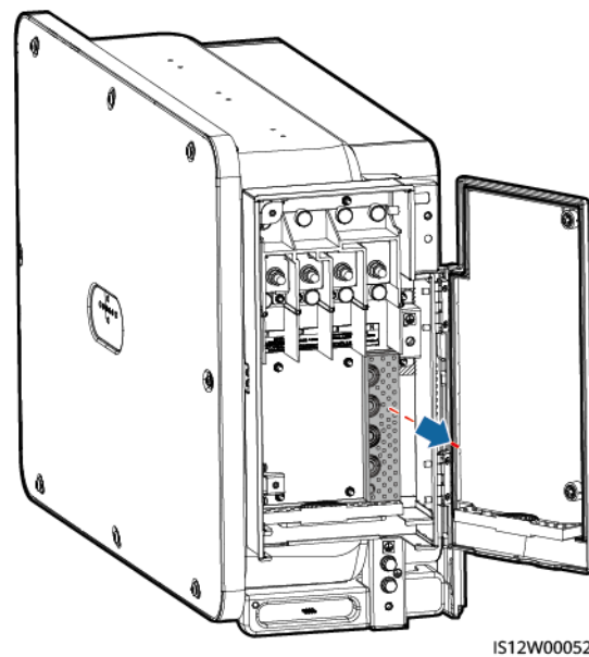
Figura 5-4 Remoção dos acessórios
