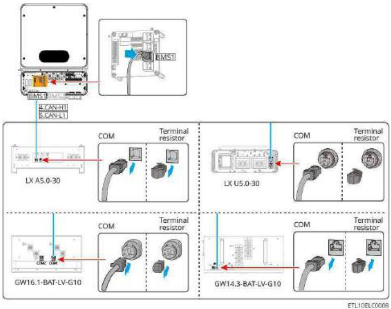
Diagrama de comunicação com ambos BMS1 e BMS2 do inversor conectados:
